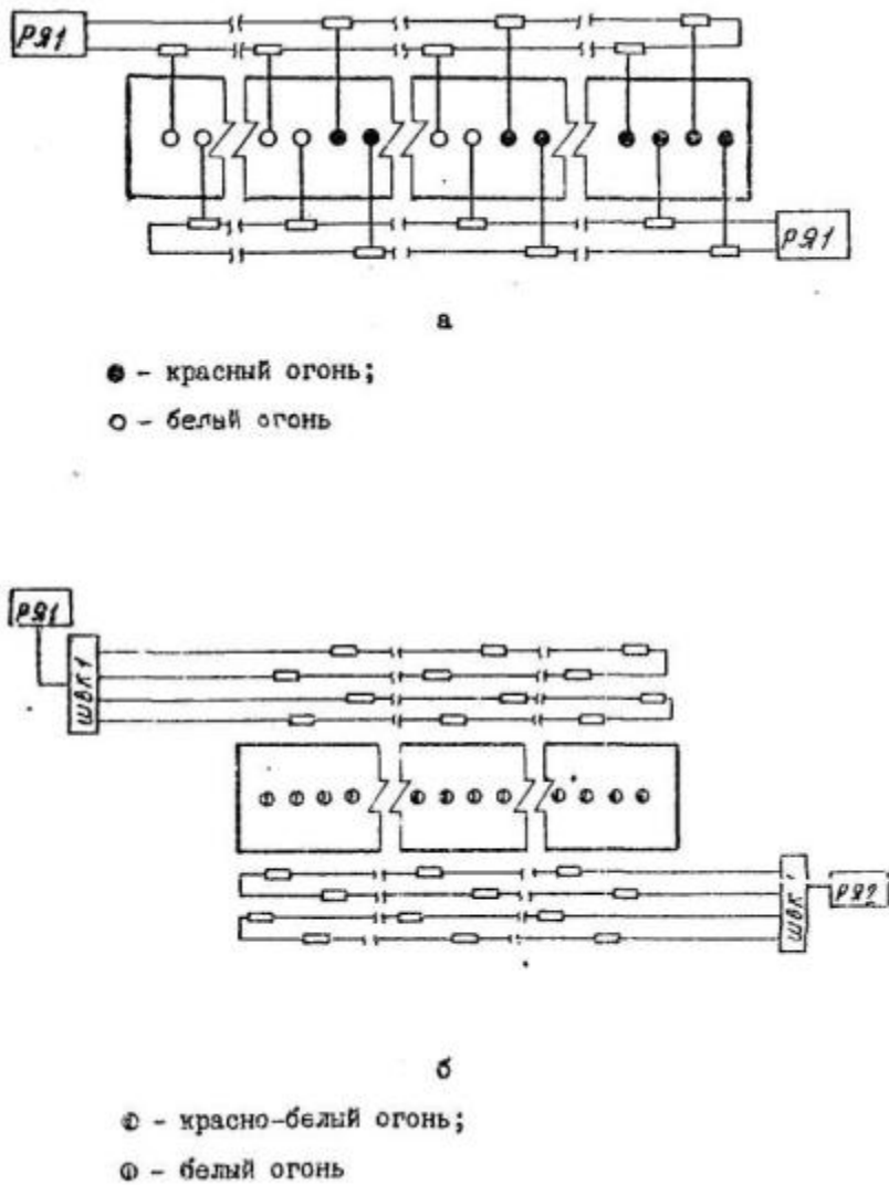
Рис. 21. Схема электропитания осевых огней ВПП: а - при установке одноламповых огней; б - при установке двухламповых огней
