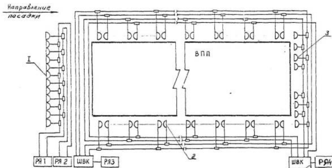
Рис. 20. Схема электропитания входных, посадочных и ограничительных огней прожекторного типа систем ОВИ-2, ОВИ-3:
