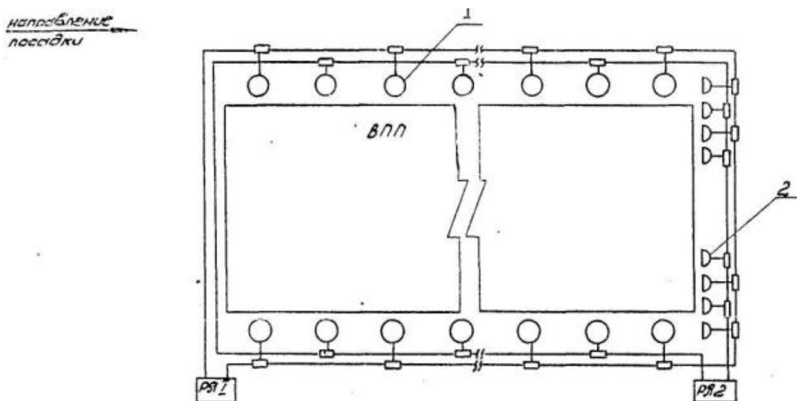
Рис. 23. Схема электропитания посадочных огней линзового типа и ограничительных огней прожекторного типа систем ОВИ-2 и ОВИ-3:
