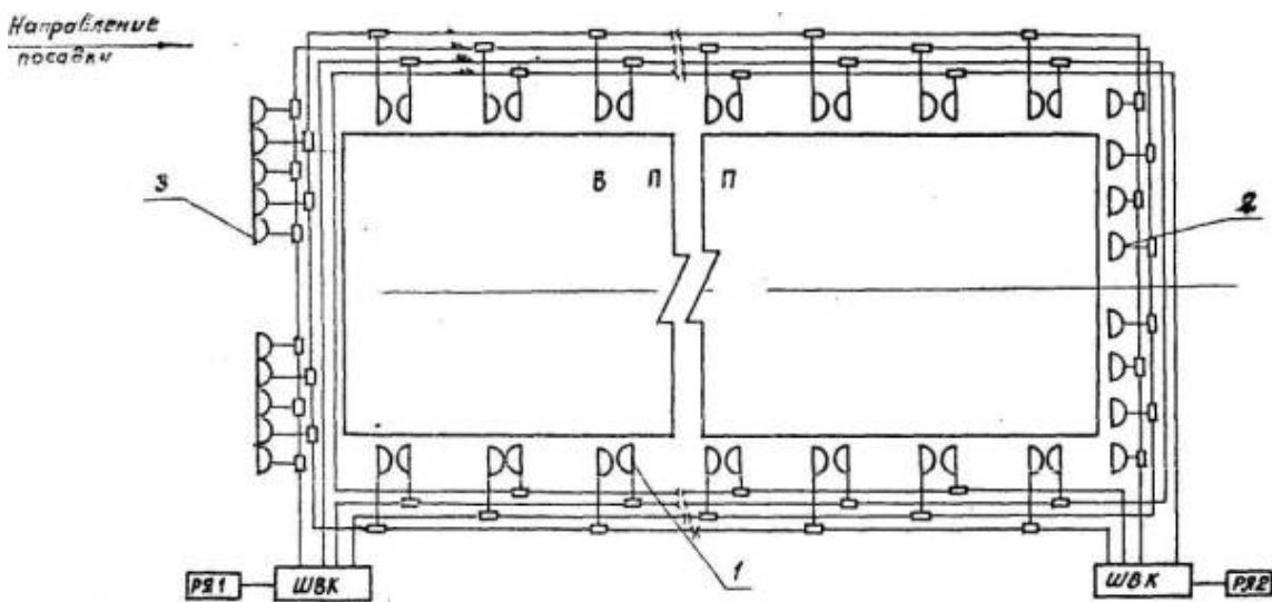
Рис. 19. Схема электропитания посадочных, входных и ограничительных огней прожекторного типа систем ОВИ-1:
