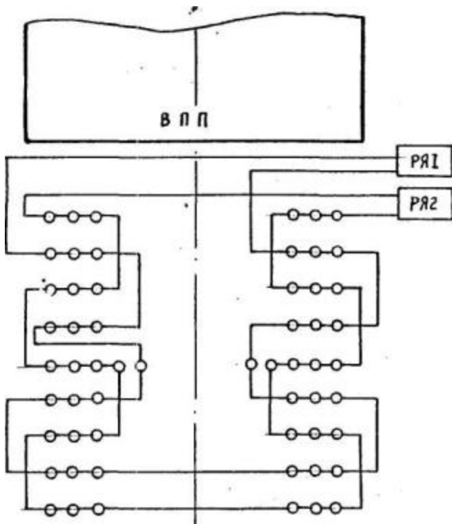
Рис. 17. Схема электропитания прожекторных боковых огней КПБ при дооборудовании системы ОВИ-1 до ОВИ-2 и ОВИ-3 с огнями приближения по центральному ряду
