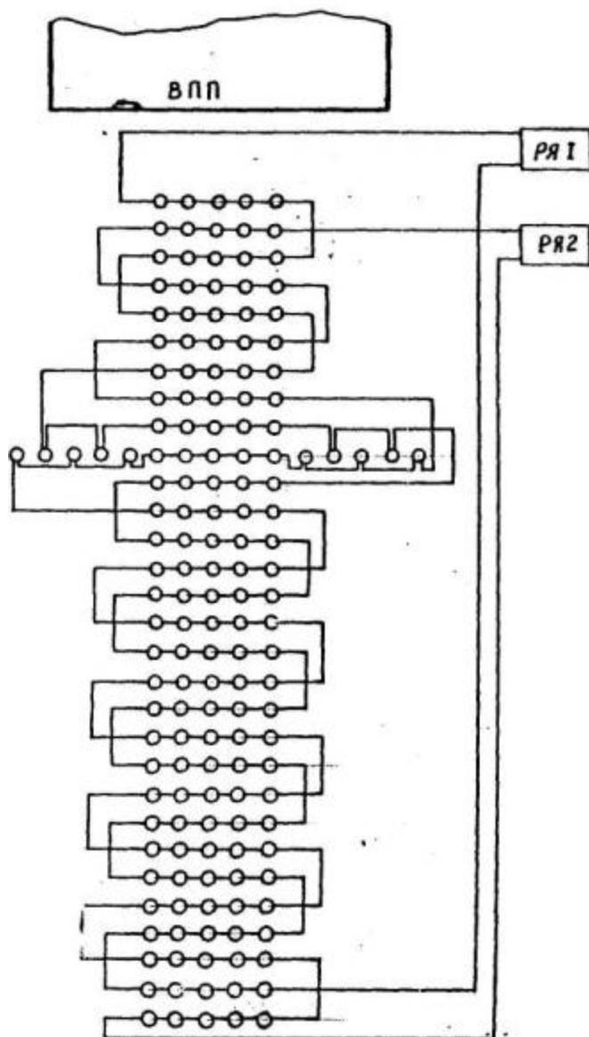
Рис. 16. Схема электропитания прожекторных огней приближения и светового горизонта систем ОВИ-1, ОВИ-2 и ОВИ-3 с огнями приближения по центральному ряду
