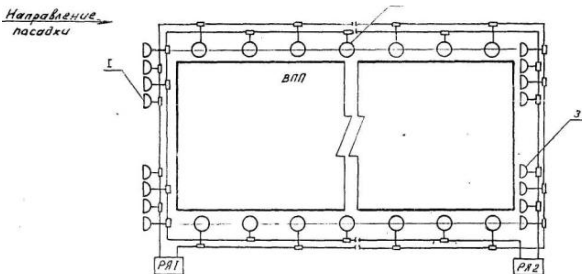
Рис. 22. Схема электропитания посадочных огней линзового типа, входных и ограничительных огней прожекторного типа систем ОВИ-1:
