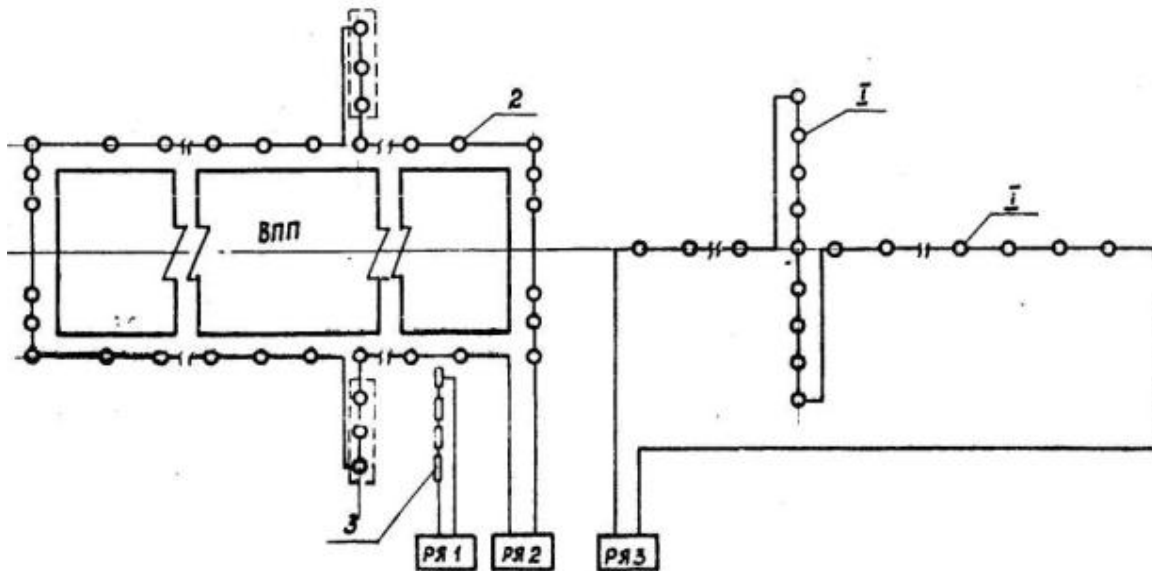
Рис. 24. Схемы электропитания огней в светосигнальных системах ОМИ:
