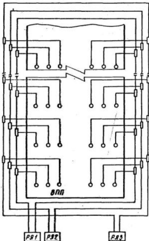
Рис. 14. Схема электропитания огней зоны приземления систем ОВИ-2 со световыми горизонтами
