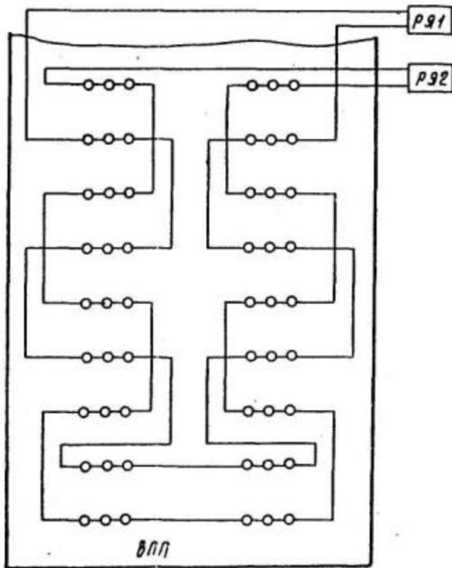
Рис. 18. Схема электропитания огней зоны приземления систем ОВИ-2, ОВИ-3 с огнями приближения по центральному ряду
