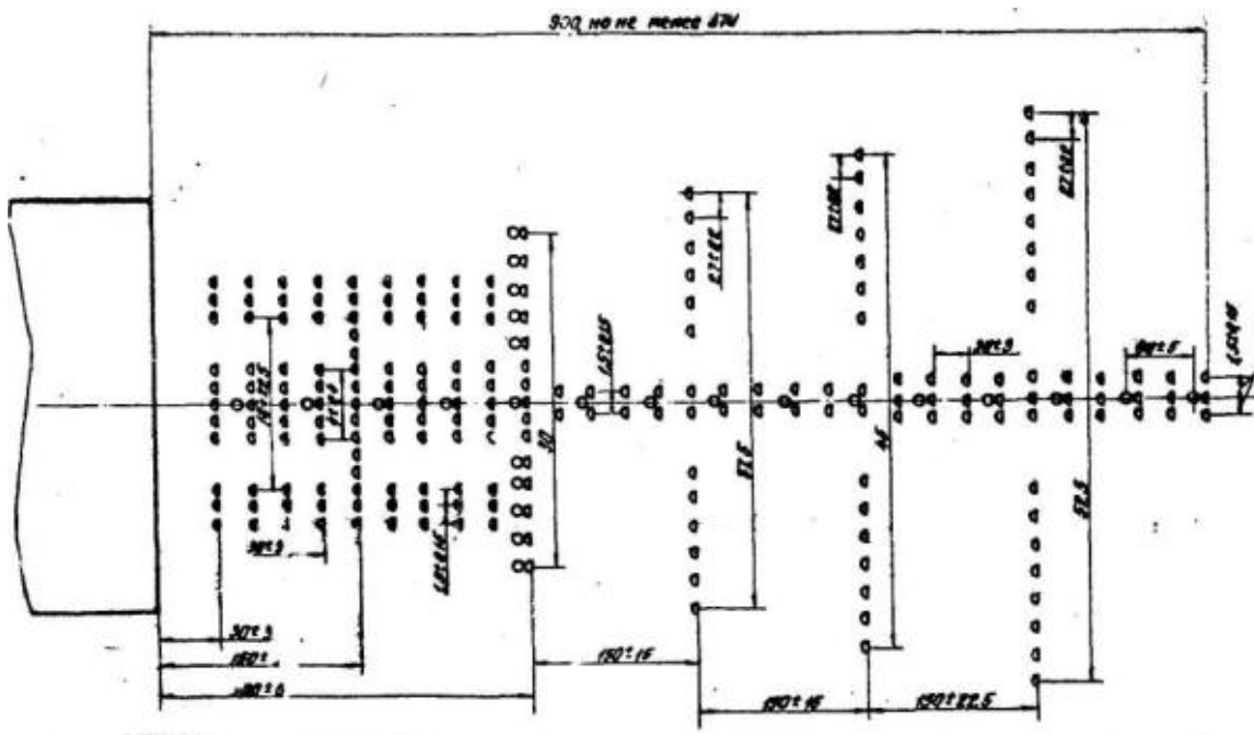
Рис. 7. Схема расположения огней приближения систем точного захода на посадку по категории II (ОВИ-2):
