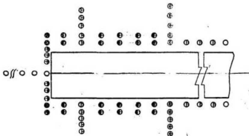
Рис. 9. Расположение светосигнального оборудования систем ОМИ при смещенном пороге:
