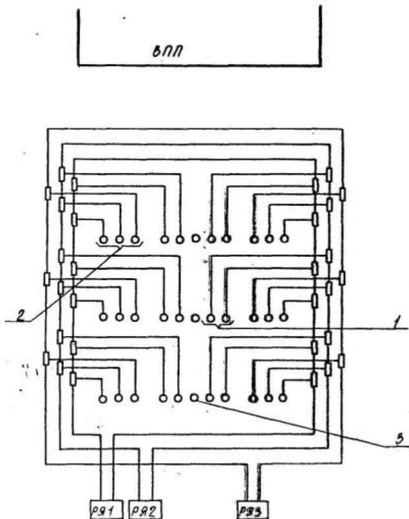
Рис. 13. Схема электропитания прожекторных огней центрального ряда и боковых огней на КПБ систем ОВИ-2 со световыми горизонтами: 1 - огни КПБ центрального ряда прожекторные; 2 - огни КПБ бокового ряда прожекторные; 3 - осевые огни КПБ прожекторные
